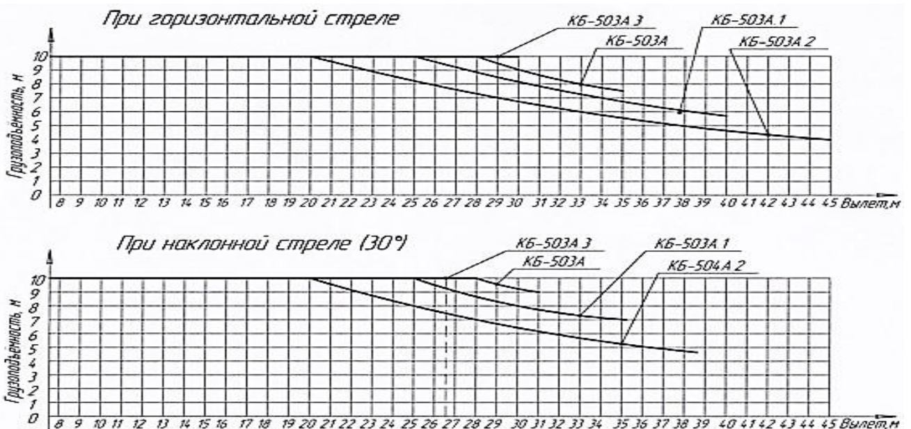
График грузоподъемности крана
